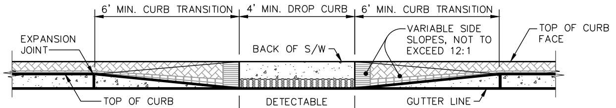
CURB ELEVATION B-B
